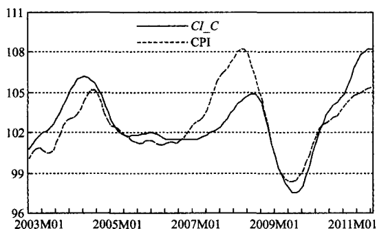
图3 购进价格合成指数 CI\_C (实线) 与 CPI (虚线)
