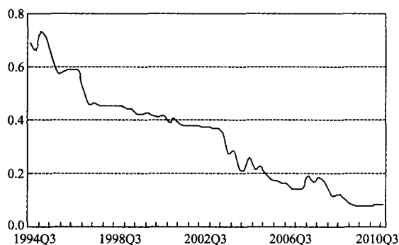
图 1 菲利普斯曲线方程中的产出缺口弹性 \beta_t
