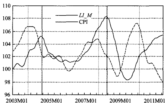
图 2 基于货币因素计算的通胀先行指数 LI\_M (虚线)与 CPI(实线)
