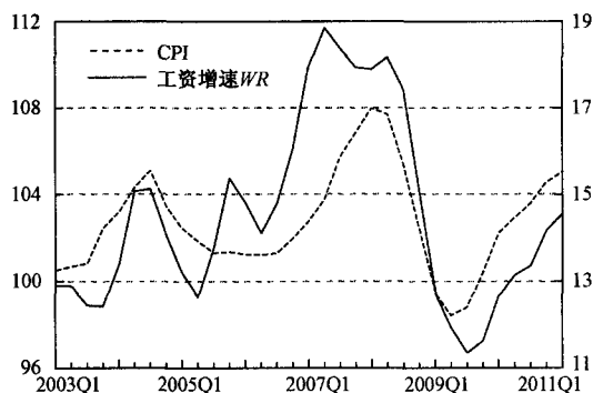
图4 工资增速 WR (实线, 右坐标) 与 CPI (虚线)
